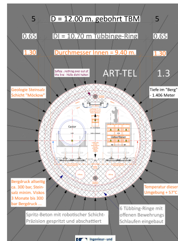
ART-TEL Schnitt Tief-Tunnel im Endlagerbereich Nov. 2017 Ing. Grottel DIN A4 in 1:100
