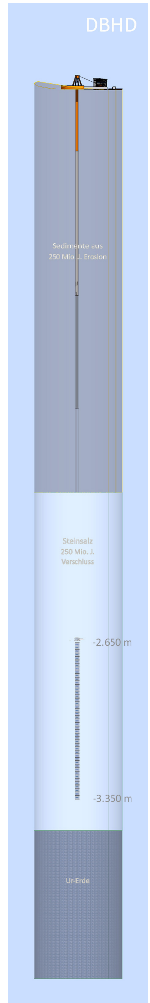
ART-TEL Schnitt Tief-Tunnel im Endlagerbereich Nov. 2017 Ing. Grottel DIN A4 in 1:100
