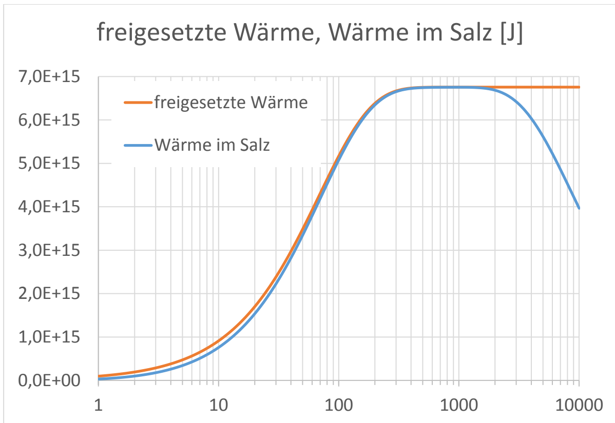
Abbildung 5: Freigesetzte Wärme in Abhängigkeit von der Zeit im Salz.
