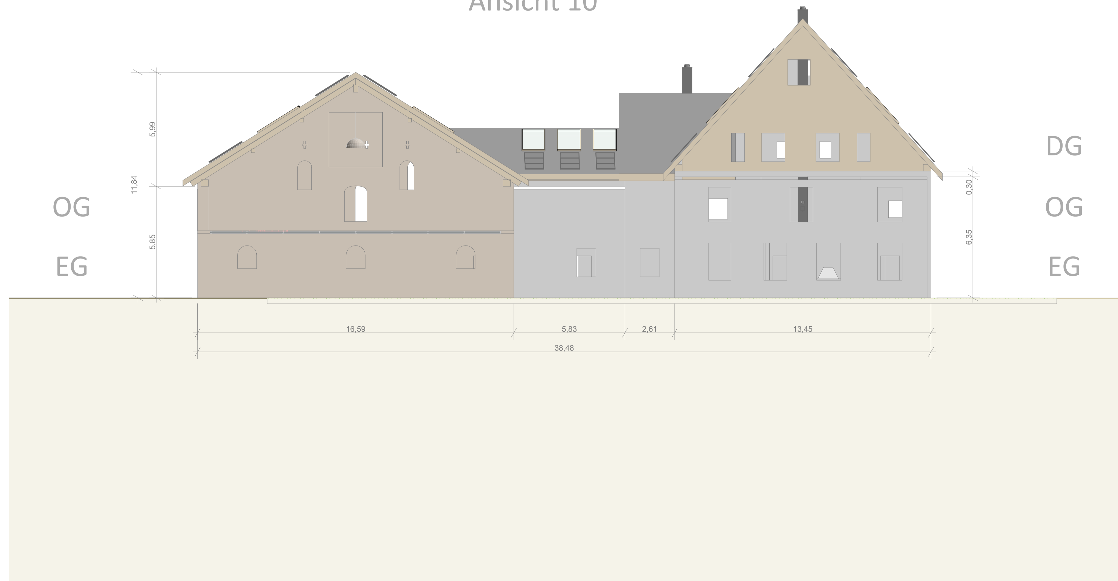
Ansicht 10
