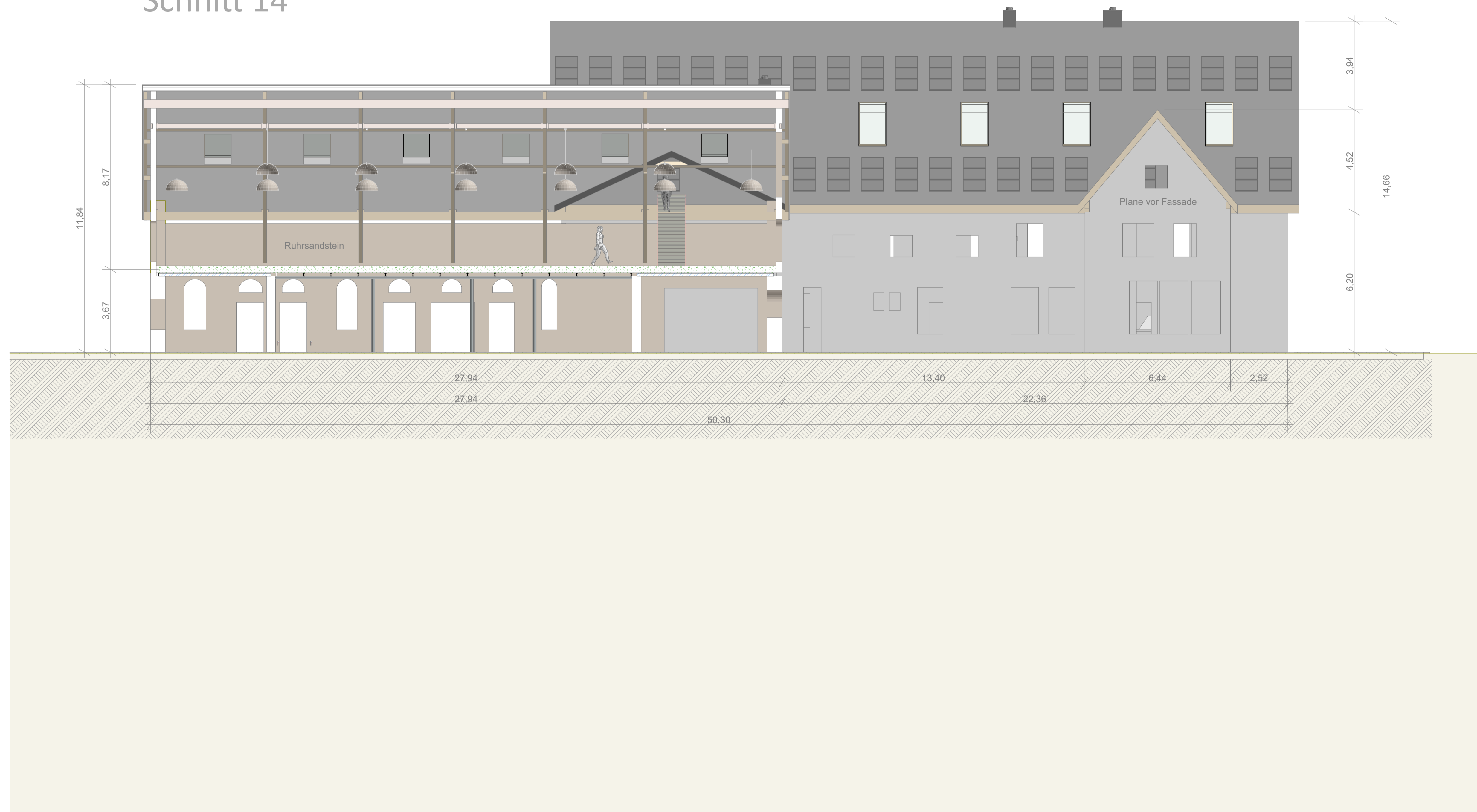
Schnitt 14
