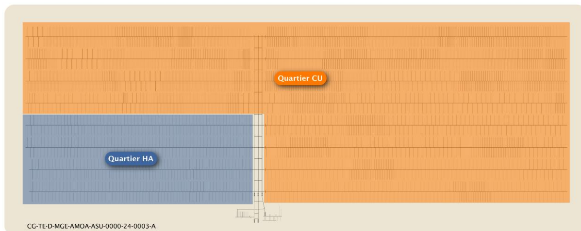
Figure 7-2 Illustration des quartiers de stockage HA et de CU (hypothèse à terminaison pour le scénario dit « SNR » enveloppe des évolutions de politique énergétique de l'Inventaire national (30))
