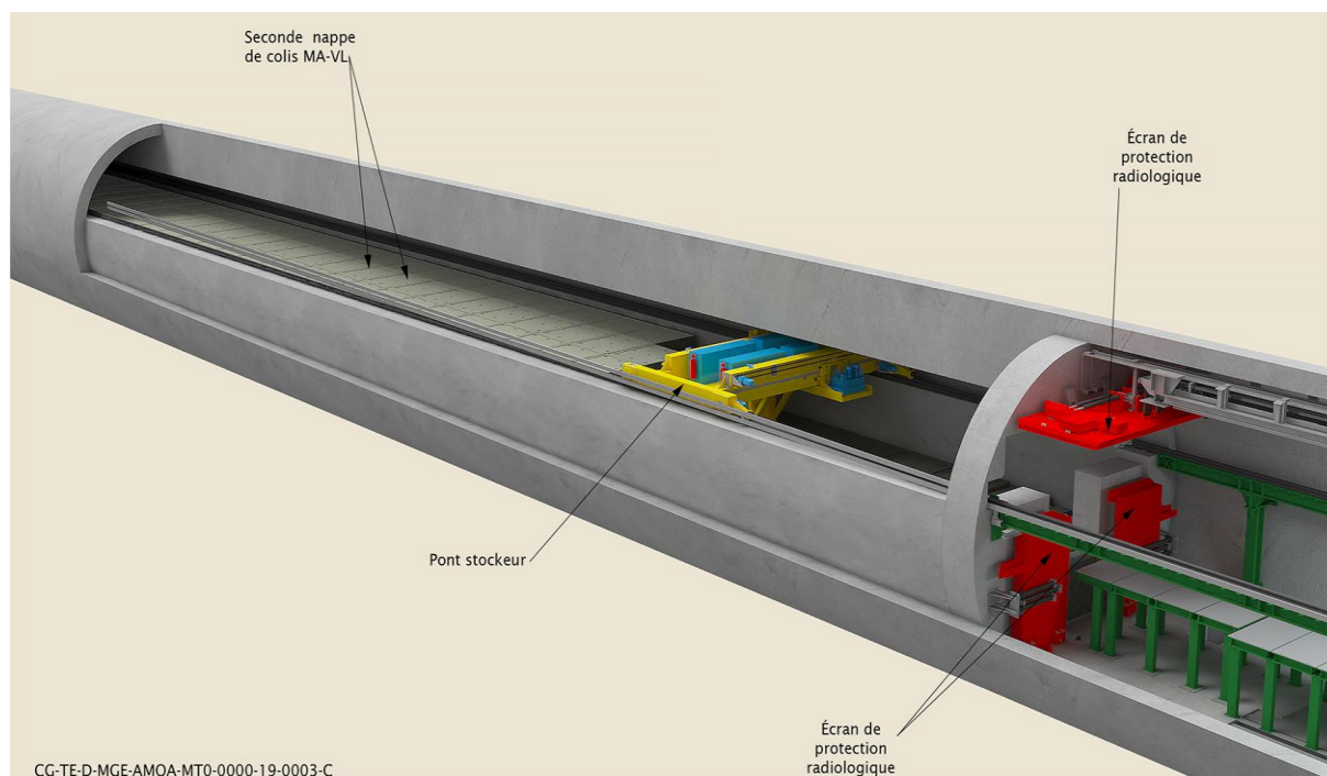
Figure Annexe 1-14 Illustration d'un alvéole MA-VL
