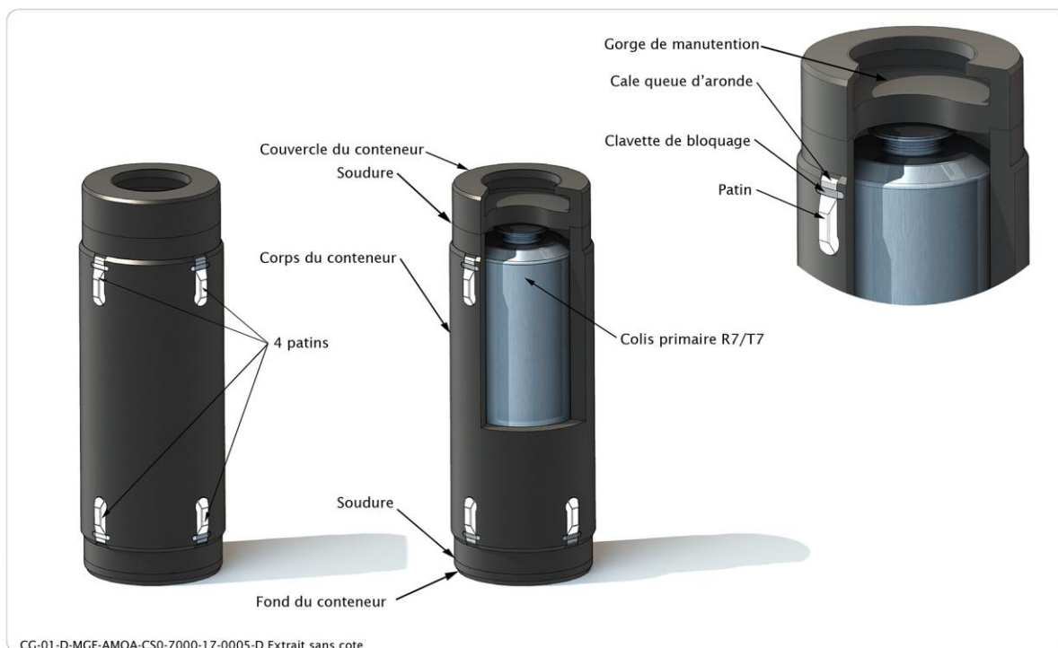
Figure Annexe 1-11 Illustration de la mise en conteneur de stockage de colis de déchets HA
