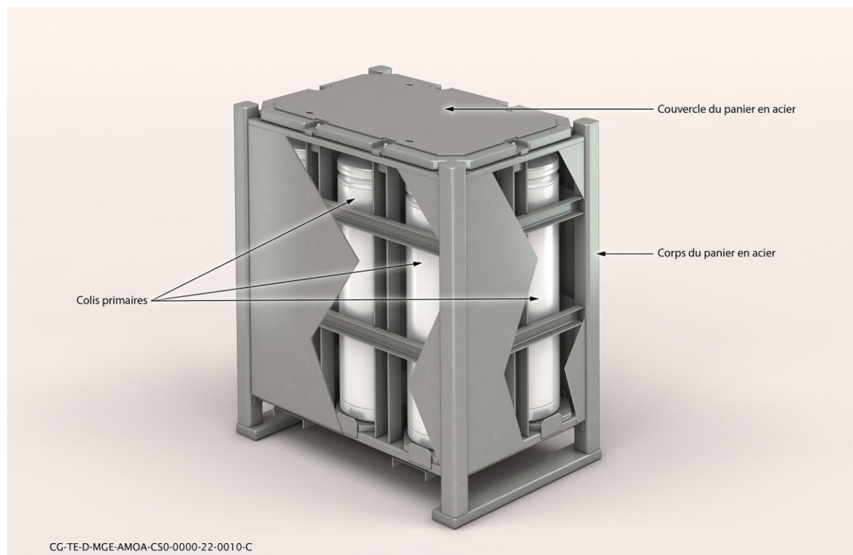
Figure Annexe 1-10 Illustration de la mise en panier de colis de déchets MA-VL
