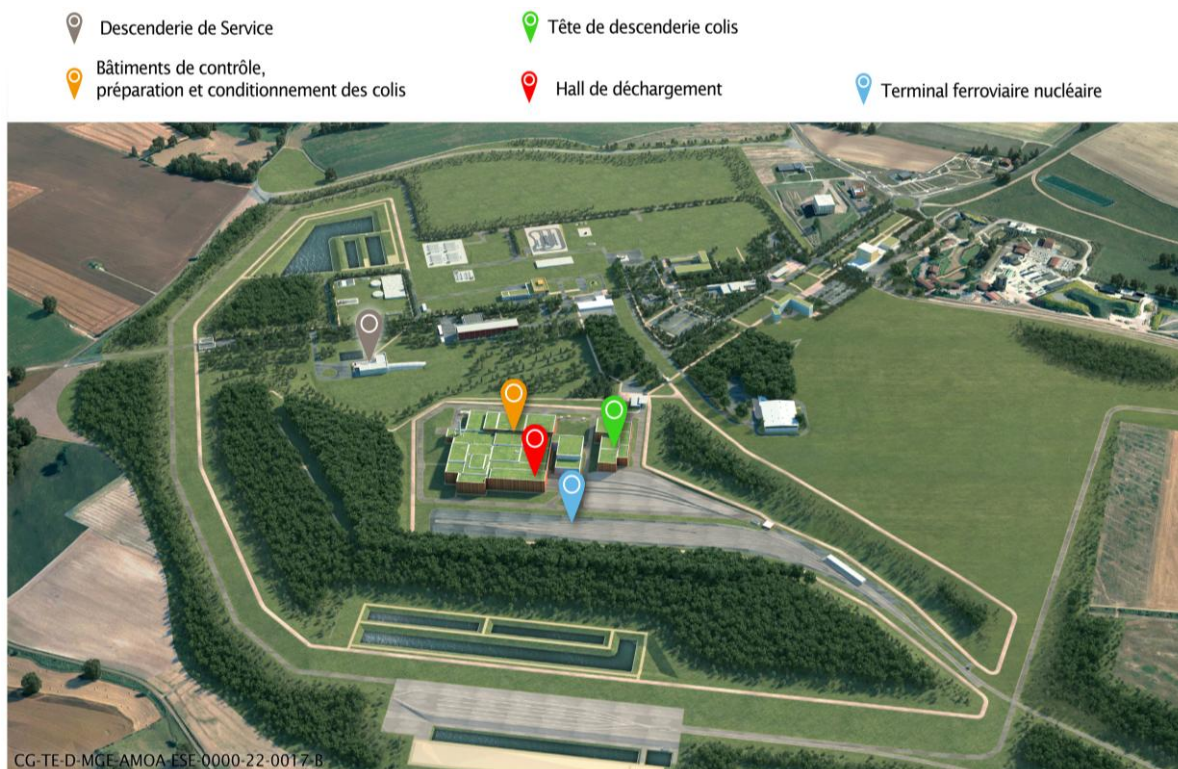
Figure 5-4 Vue illustrative des ouvrages de la zone descenderie construits pendant la phase de construction initiale (Espace technologique et Laboratoire souterrain préexistants représentés à titre indicatif)
