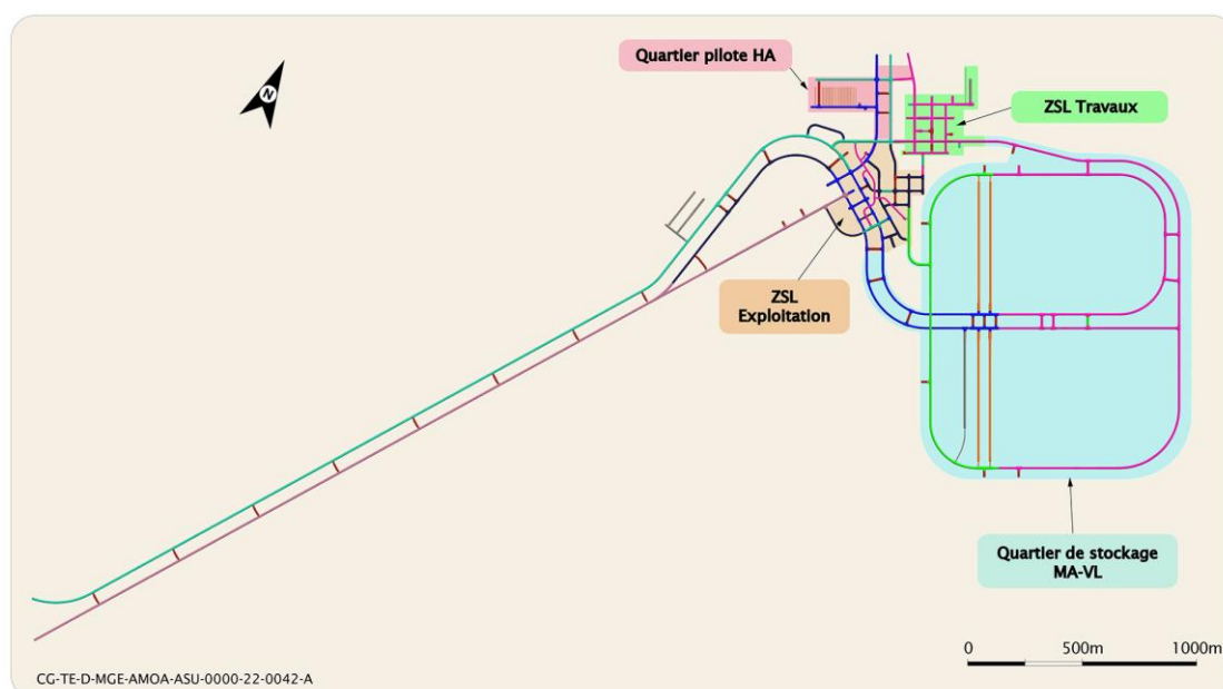
Figure 5-3 Illustration des ouvrages souterrains construits lors de la phase de construction initiale
